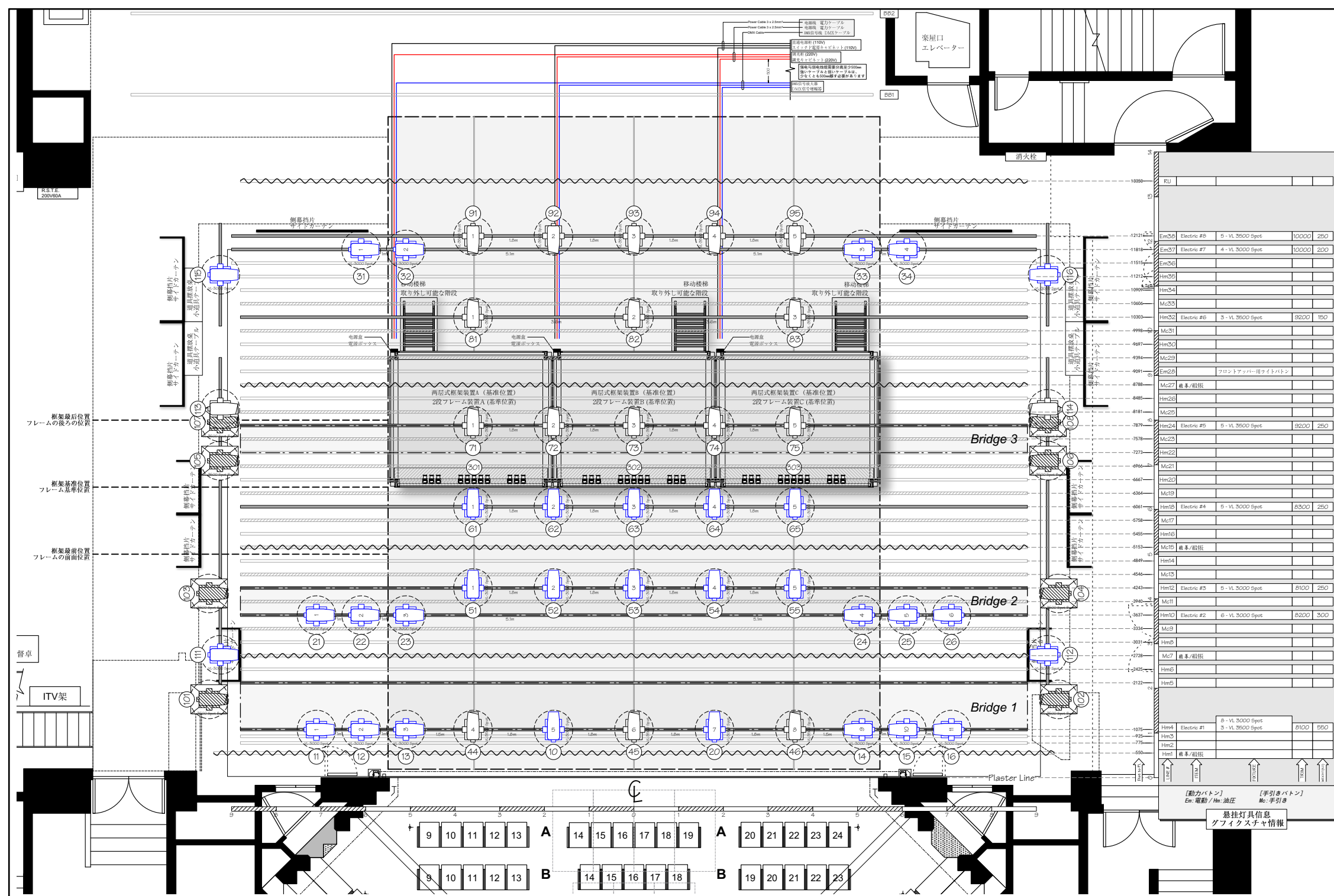
1 舞台区域灯位图 ステージエリアライトプロット Scale 1:100 / A3
